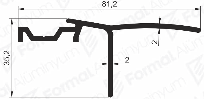
Pr.No: 8584 0,721 kg/m
