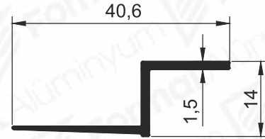
Pr.No: 9562 0,243 kg/m
