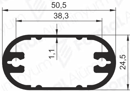
Pr.No: 9568 0,778 kg/m
