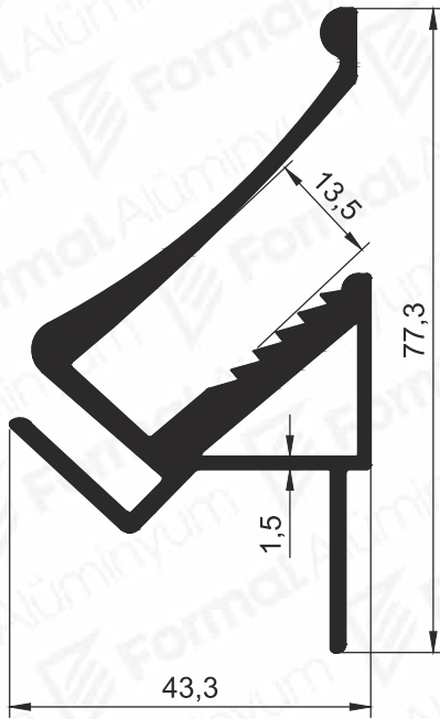
Pr.No: 8691 1,450 kg/m
