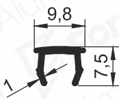
Pr.No: 1035 0,065 kg/m
