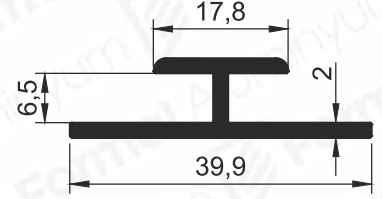
Pr.No: 9246 0,345 kg/m
