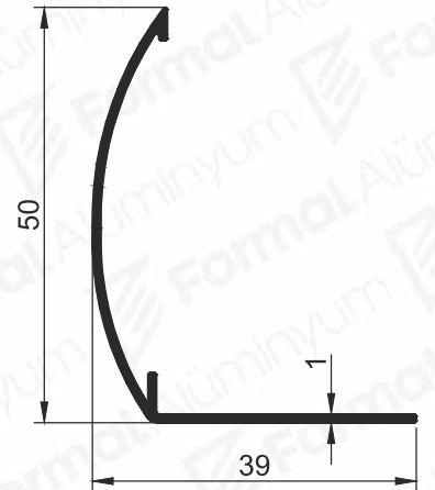
Pr.No: 8598 0,247 kg/m
