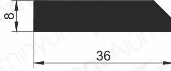
Pr.No: 9118 0,746 kg/m
