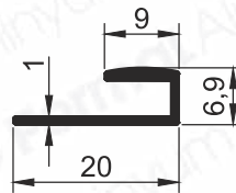
Pr.No: 1126 0,099 kg/m
