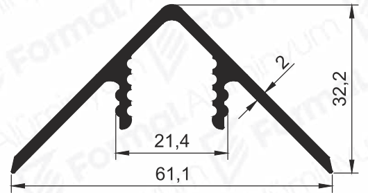
Pr.No: 8645 0,614 kg/m
