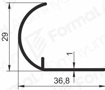
Pr.No: 1544 0,195 kg/m
