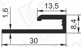
Pr.No: 8669 0,223 kg/m
