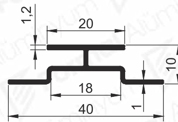
Pr.No: 4709 0,205 kg/m
