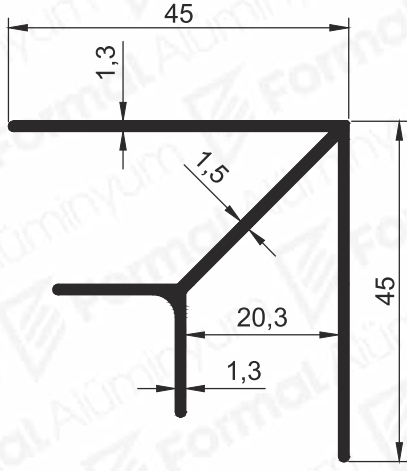
Pr.No: 1111 0,551 kg/m
