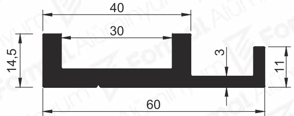
Pr.No: 8660 1,024 kg/m
