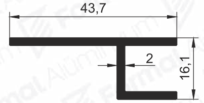
Pr.No: 9002 0,384 kg/m
