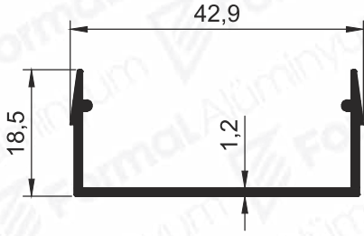
Pr.No: 8588 0,263 kg/m
