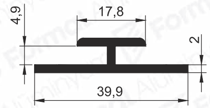
Pr.No: 8508 0,334 kg/m
