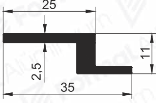
Pr.No: 9117 0,339 kg/m
