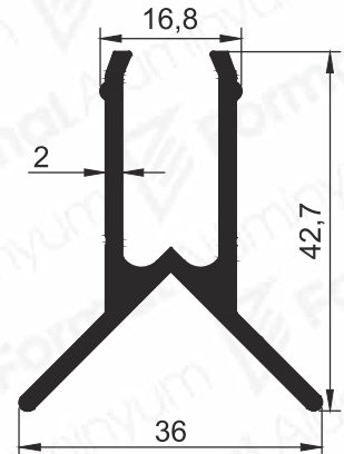
Pr.No: 8646 0,635 kg/m
