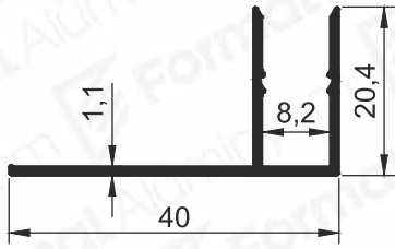
Pr.No: 1105 0,233 kg/m
