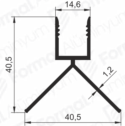
Pr.No: 1107 0,352 kg/m
