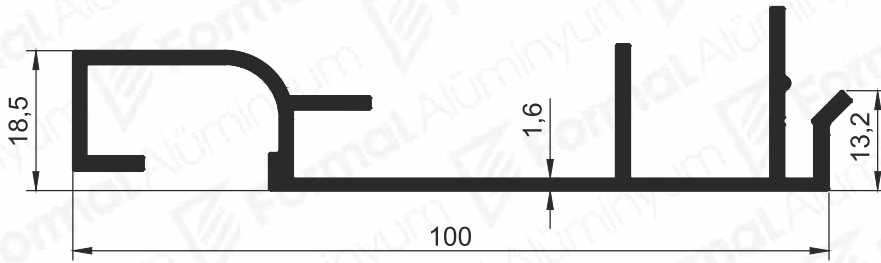
Pr.No: 8913 0,93 kg/m
