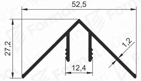
Pr.No: 1106 0,330 kg/m
