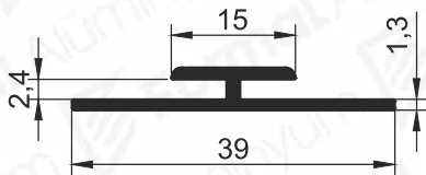
Pr.No: 8963 0,206 kg/m
