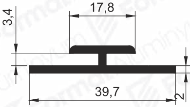
Pr.No: 8507 0,339 kg/m
