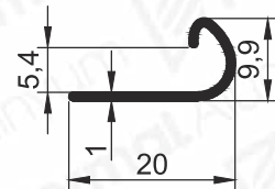
Pr.No: 8633 0,085 kg/m
