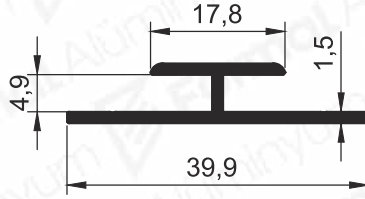
Pr.No: 1545 0,251 kg/m
