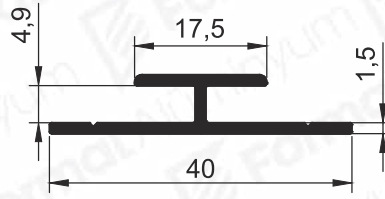
Pr.No: 2157 0,243 kg/m
