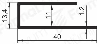
Pr.No: 8676 0,263 kg/m
