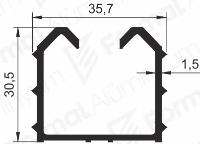
Pr.No: 8644 0,479 kg/m
