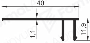
Pr.No: 1104 0,186 kg/m
