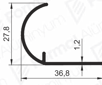
Pr.No: 8539 0,218kg/m
