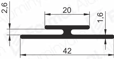
Pr.No: 8708 0,289 kg/m
