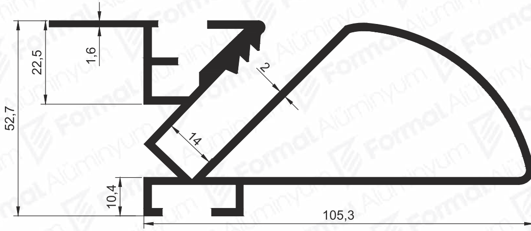
Pr.No: 8912 2,245 kg/m
