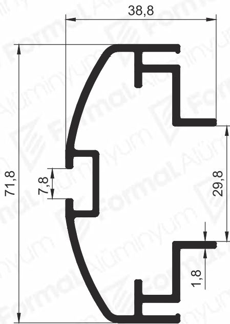
Pr.No: 8910 1,024 kg/m
