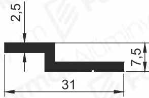
Pr.No: 9562 0,243 kg/m
