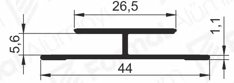
Pr.No: 9946 0,227 kg/m
