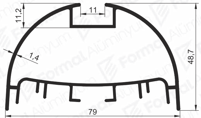
Pr.No: 8962 1,023 kg/m
