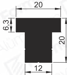
Pr.No: 9767 0,785 kg/m
