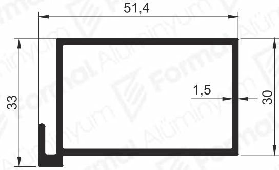
Pr.No: 8626 0,685 kg/m
