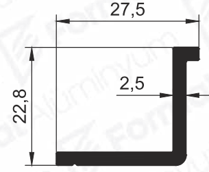
Pr.No: 9119 0,321 kg/m
