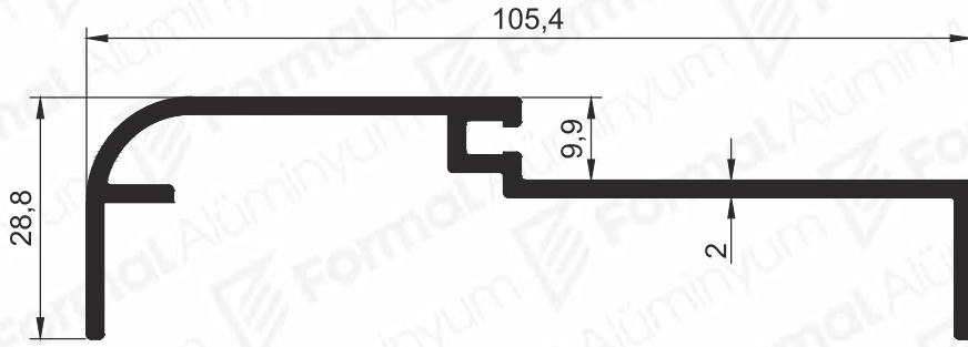
Pr.No: 8839 0,932 kg/m
