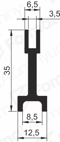
Pr.No: 8562 0,400 kg/m
