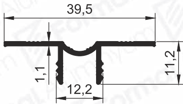
Pr.No: 1109 0,187 kg/m
