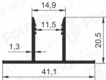
Pr.No: 1108 0,258 kg/m
